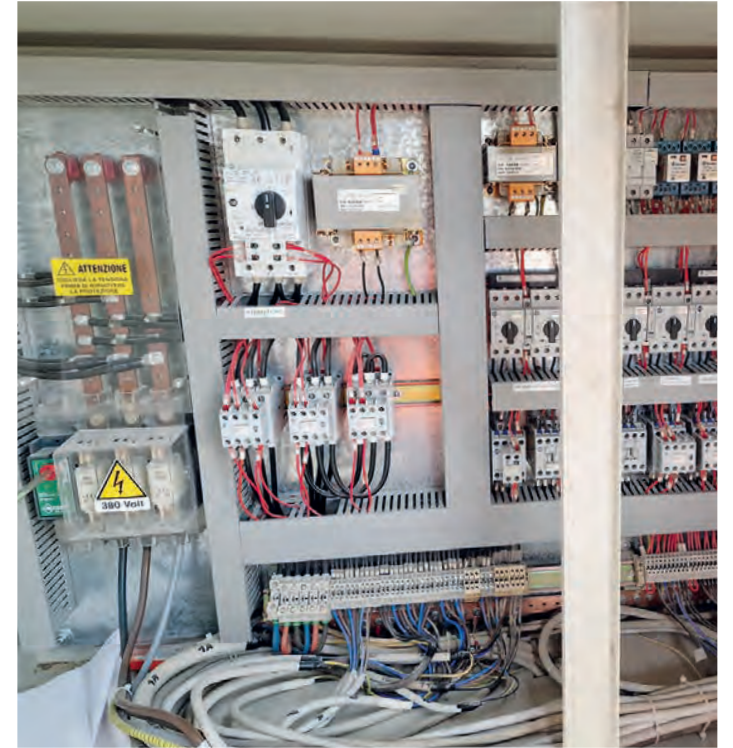
QUADRO COMANDO
